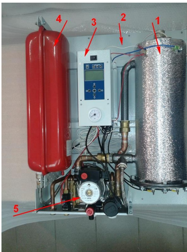
Рисунок 2. Общий вид водонагревателя «Premium Plus»
