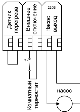
Рисунок 5. Колодка подключения внешнего оборудования
