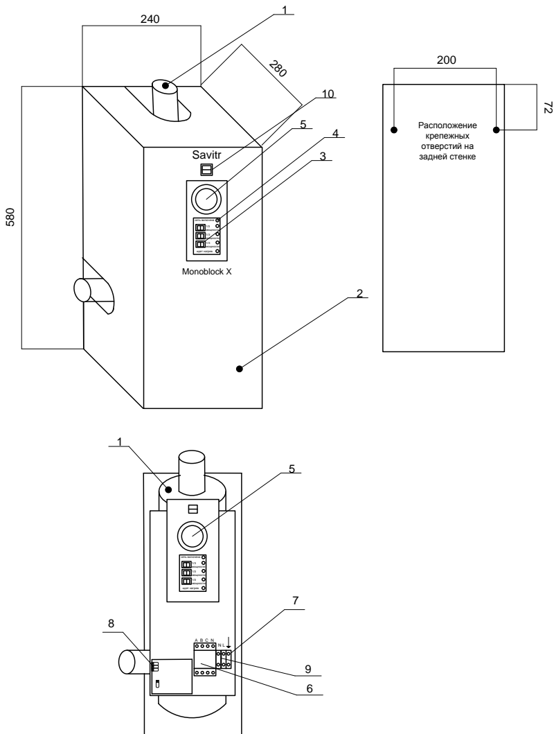
Рис.1 Общий вид изделия типа «Monoblock X».
