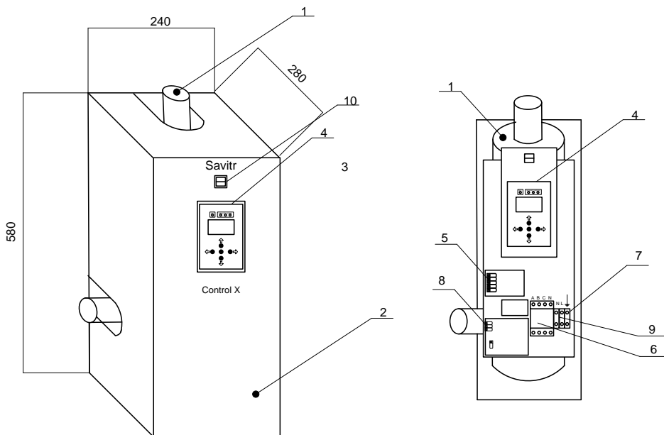
Рис.2 Общий вид изделия модели «Control X».
