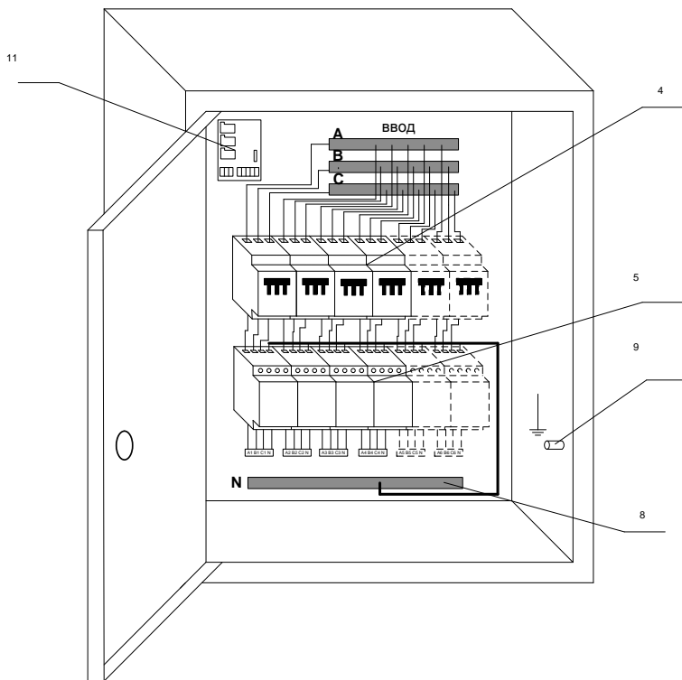
Рис. 1б. Внешний вид изделия типа Savitr «Prof X» (60-144 кВт).
