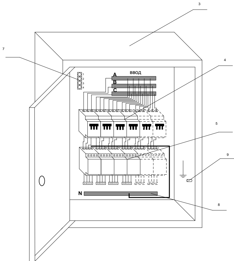
Рис. 1а. Внешний вид изделия типа Savitr «Max X» (60-144 кВт).
